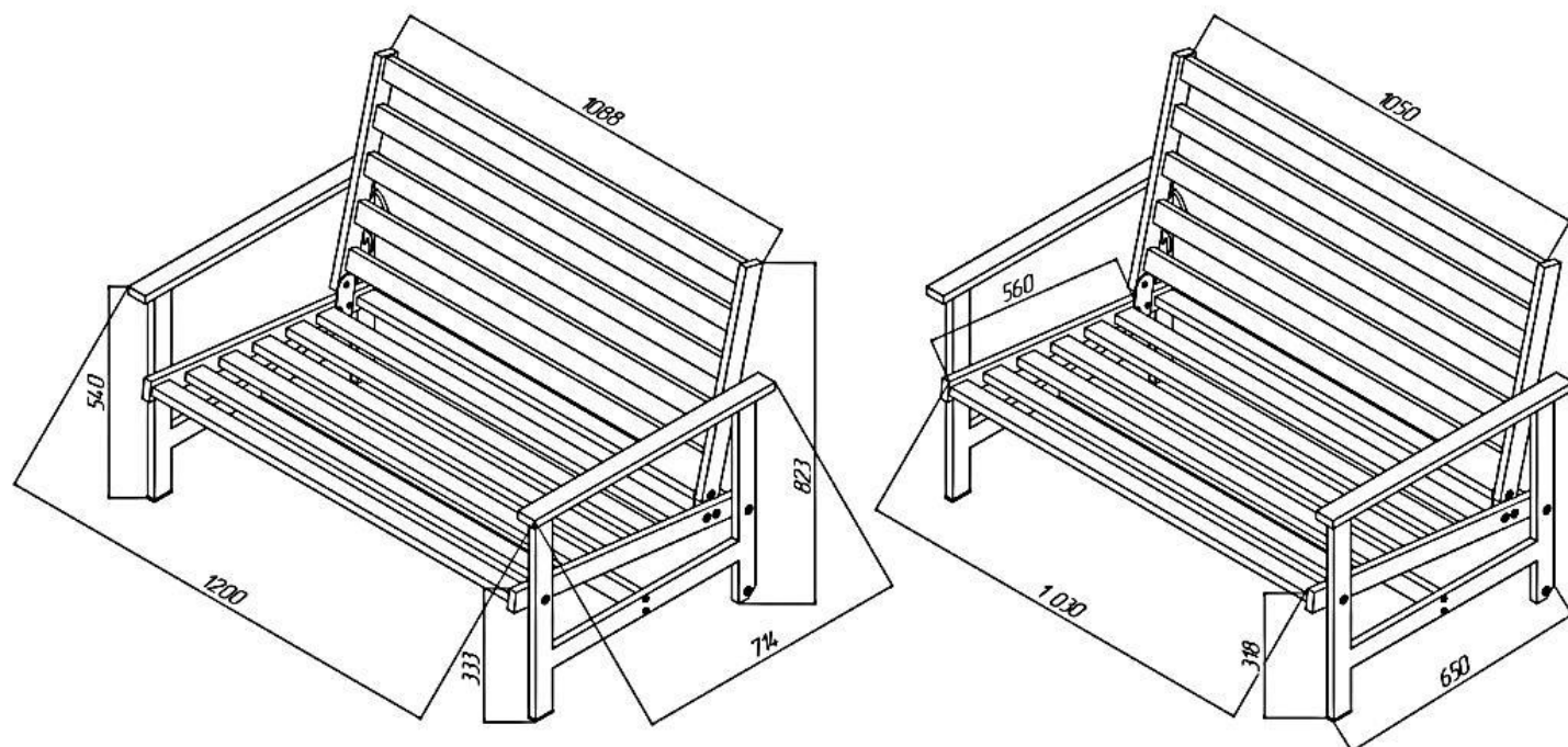
Рисунок 2 – Диван двухместный SKL.01.0103.03. Общий вид и габаритные размеры, мм
