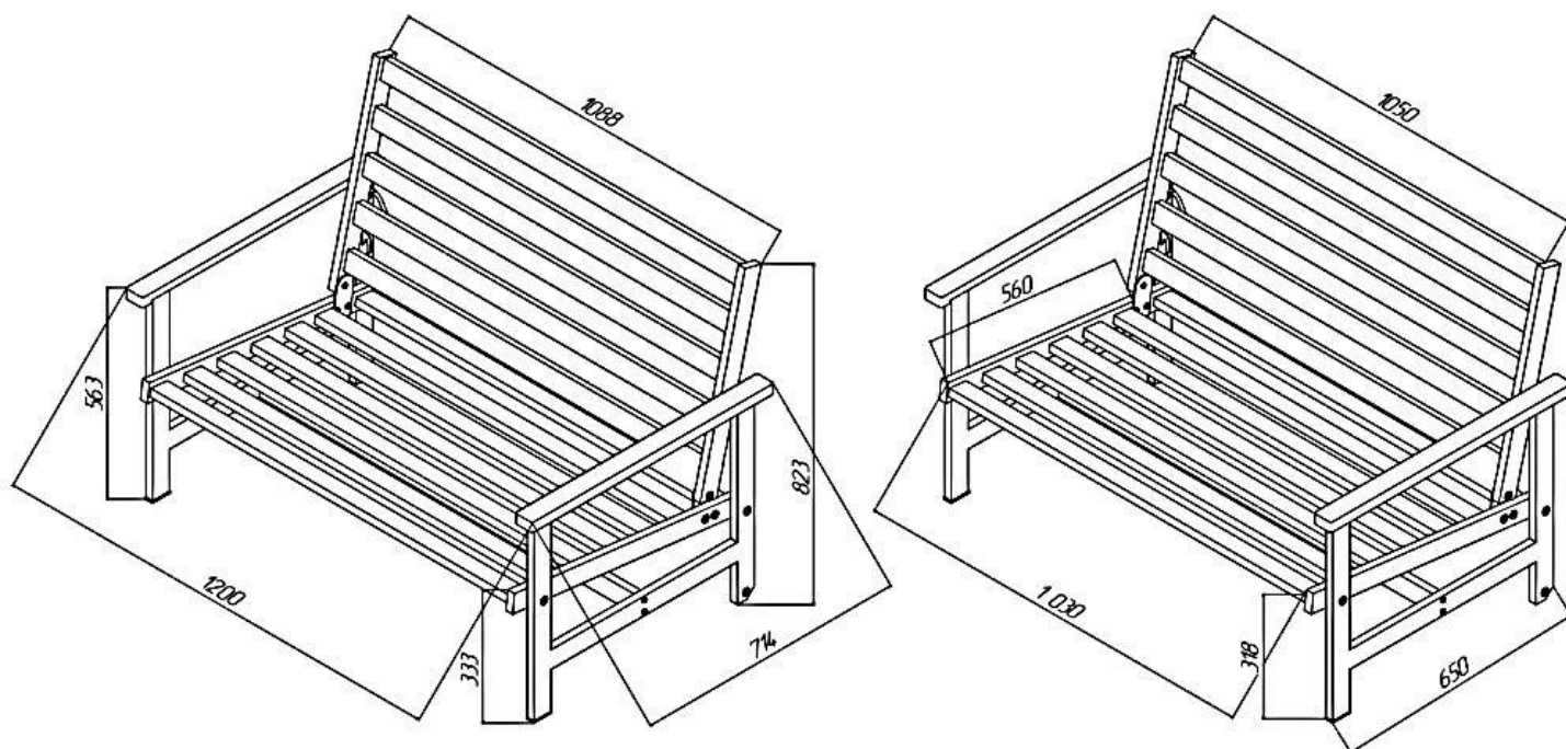
Рисунок 1 – Диван двухместный с деревянным подлокотником SKL.01.0103.01. Общий вид и габаритные размеры, мм
