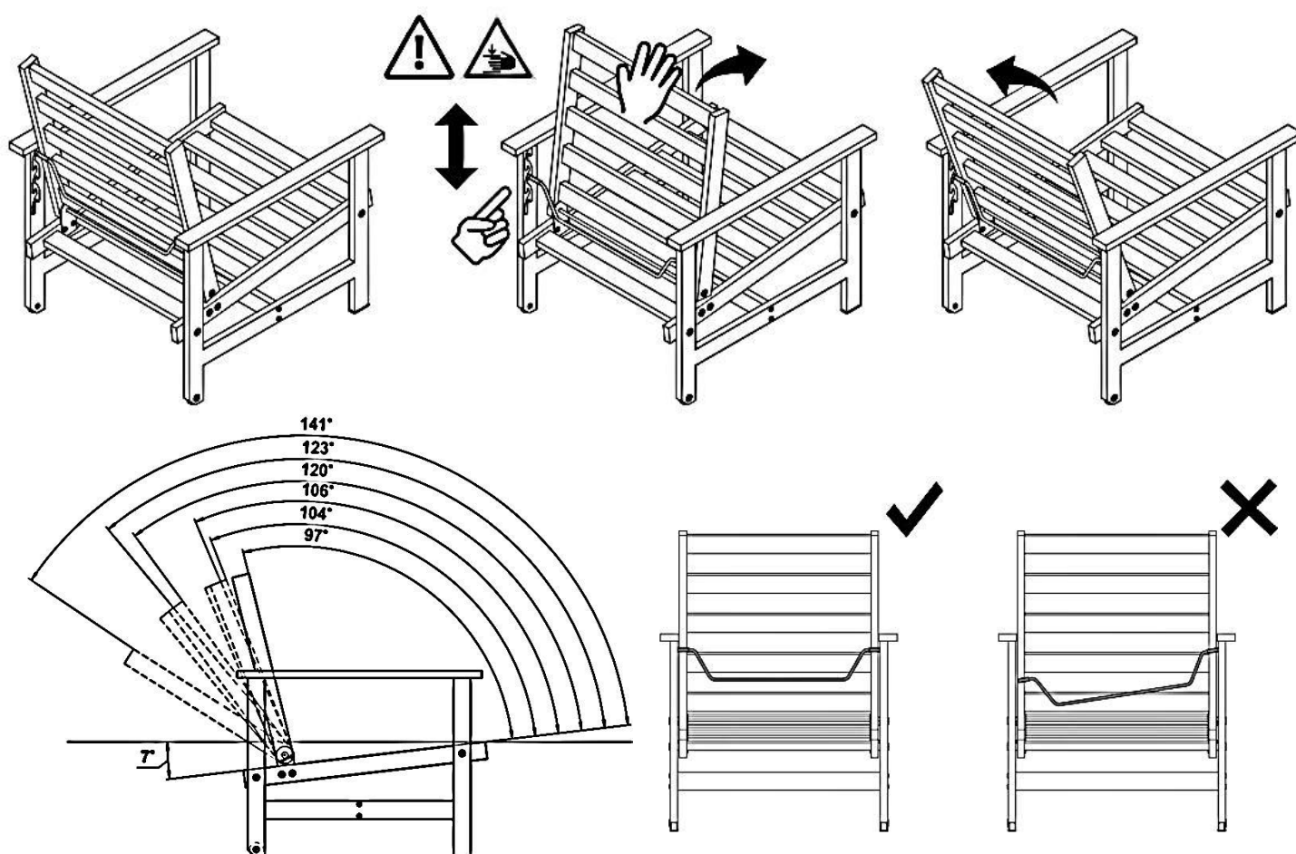
Рисунок 3 - Схема регулировки спинки изделий
