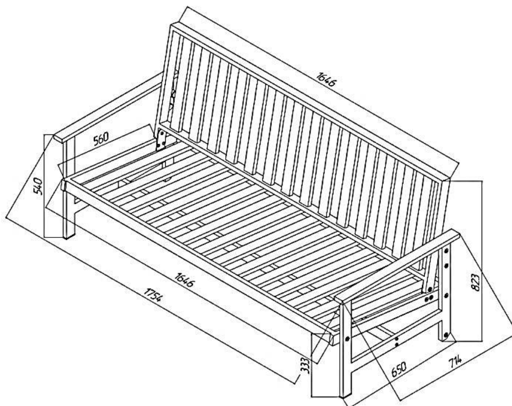
Рисунок 2 – Диван SKL.01.0103.04. Общий вид и габаритные размеры, мм
