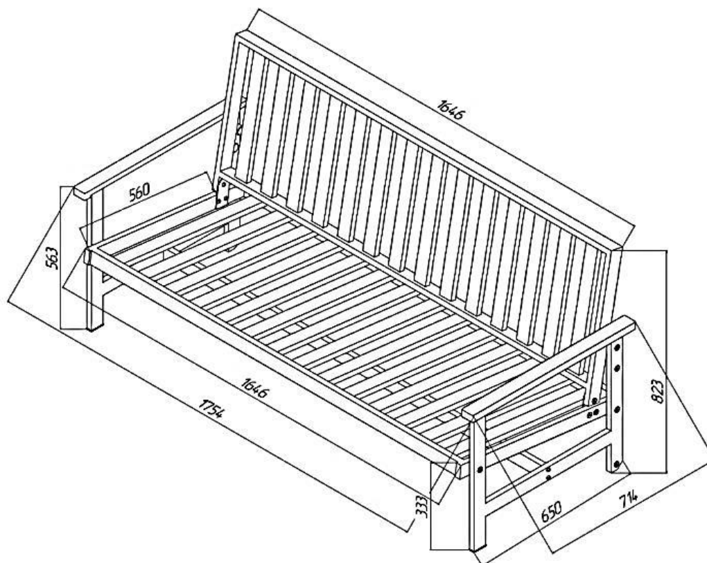
Рисунок 1 – Диван с деревянным подлокотником SKL.01.0103.02. Общий вид и габаритные размеры, мм
