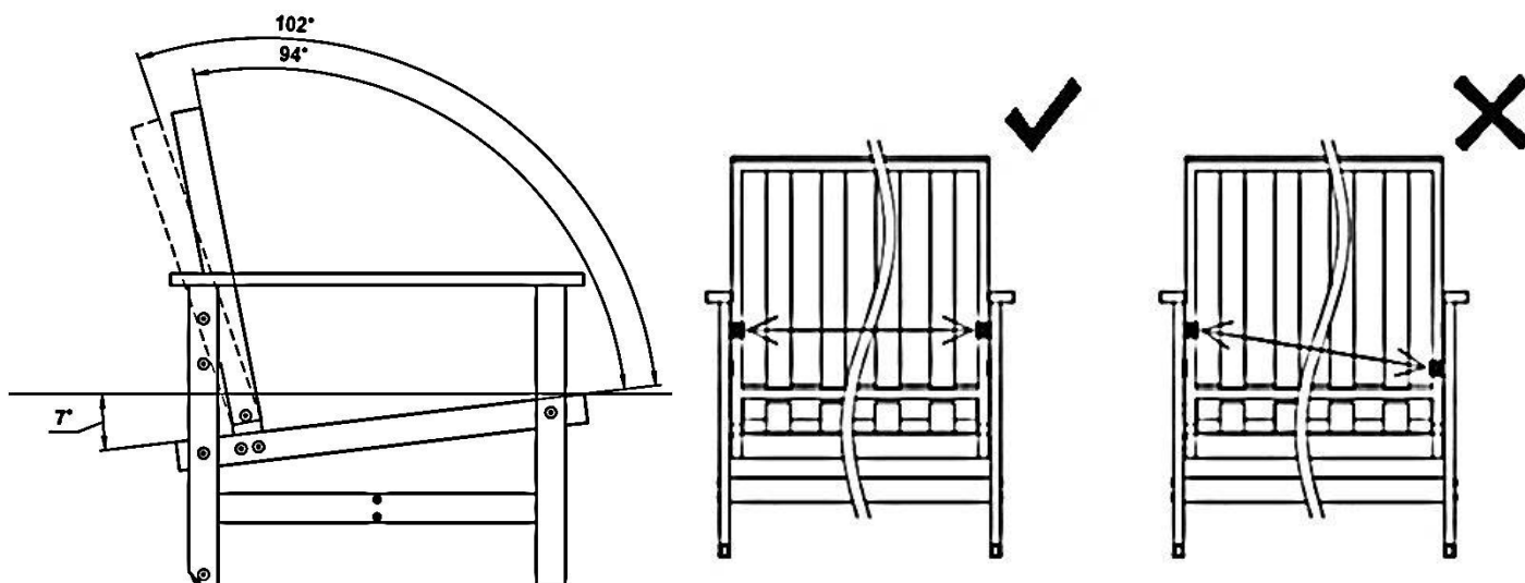
Рисунок 3 - Схема регулировки спинки изделий
