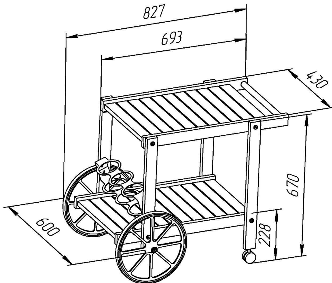
Рисунок 1 – Стол сервировочный SKL.01.0106.03. Общий вид и габаритные размеры, мм
