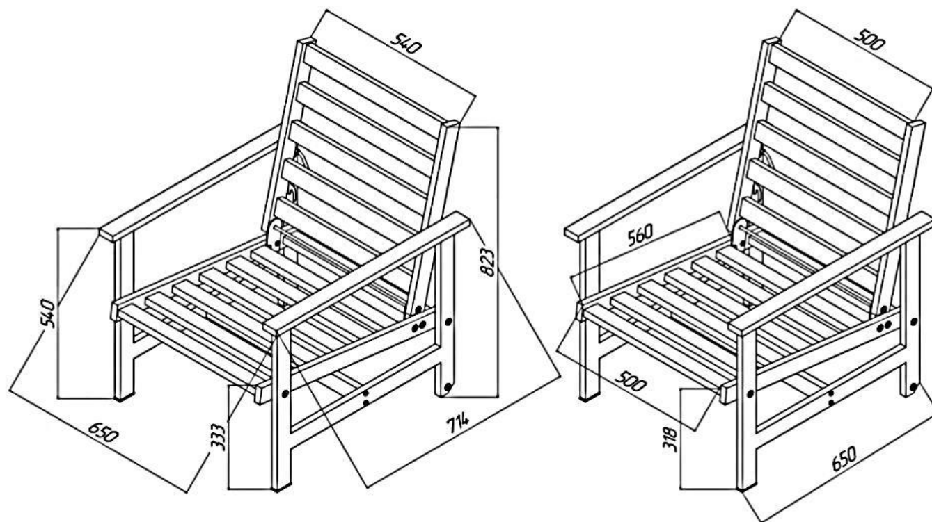
Рисунок 2 – Кресло SKL.01.0101.02. Общий вид и габаритные размеры, мм
