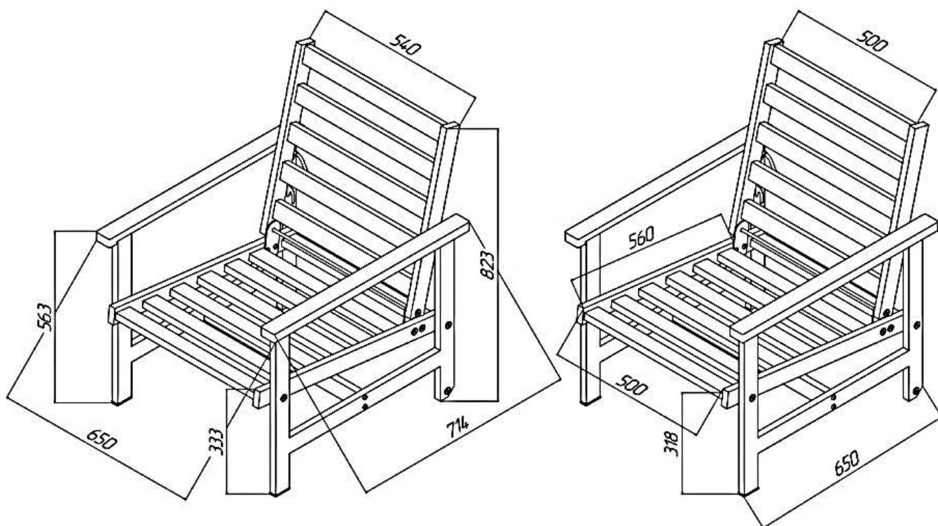
Рисунок 1 – Кресло с деревянным подлокотником SKL.01.0101.01. Общий вид и габаритные размеры, мм
