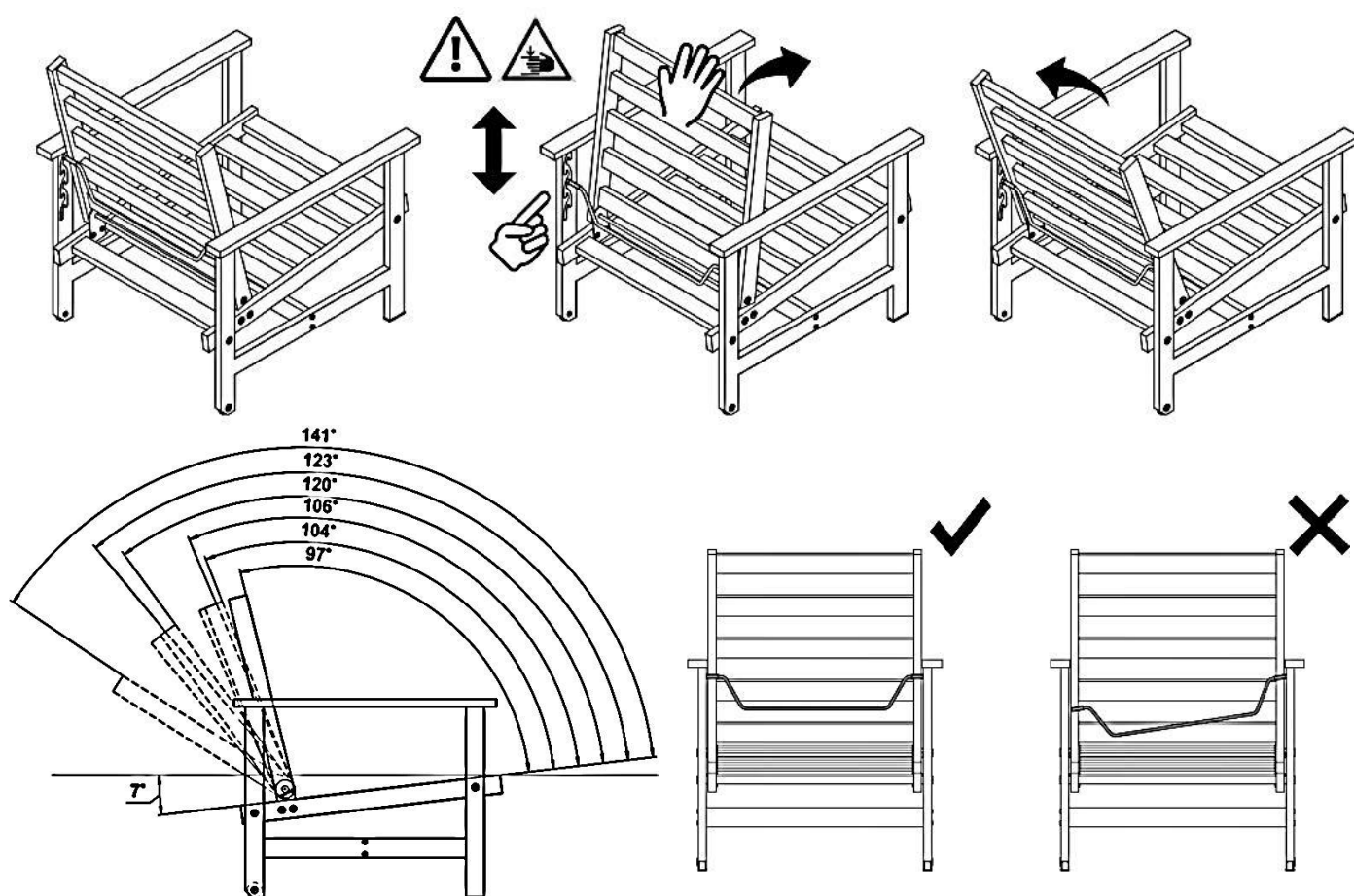
Рисунок 3 - Схема регулировки спинки изделий
