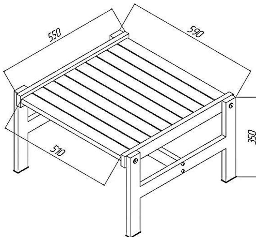
Рисунок 1 – Банкетка SKL.01.0107.01. Общий вид и габаритные размеры, мм
