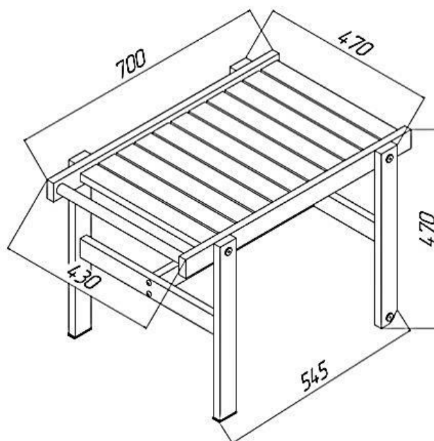
Рисунок 1 – Стол подкатной SKL.01.0106.04. Общий вид и габаритные размеры, мм
