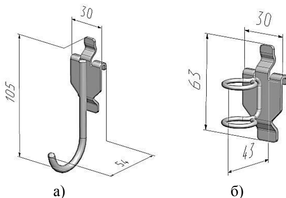
Рисунок 1 – Общий вид и габаритные размеры изделий, мм: а) крюк J-образный REL.01.0202.01; б) крюк для отверток REL.01.0202.02.
