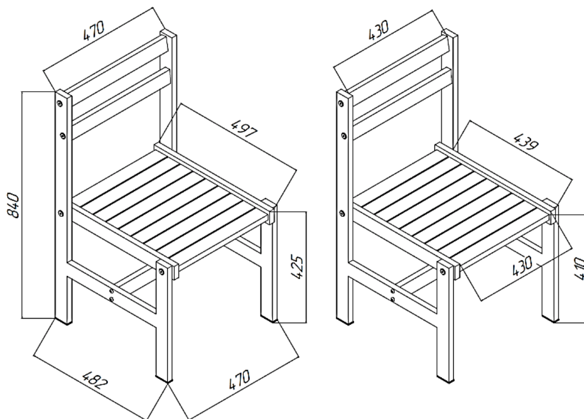
Рисунок 1 – Стул SKL.01.0102.01. Общий вид и габаритные размеры, мм
