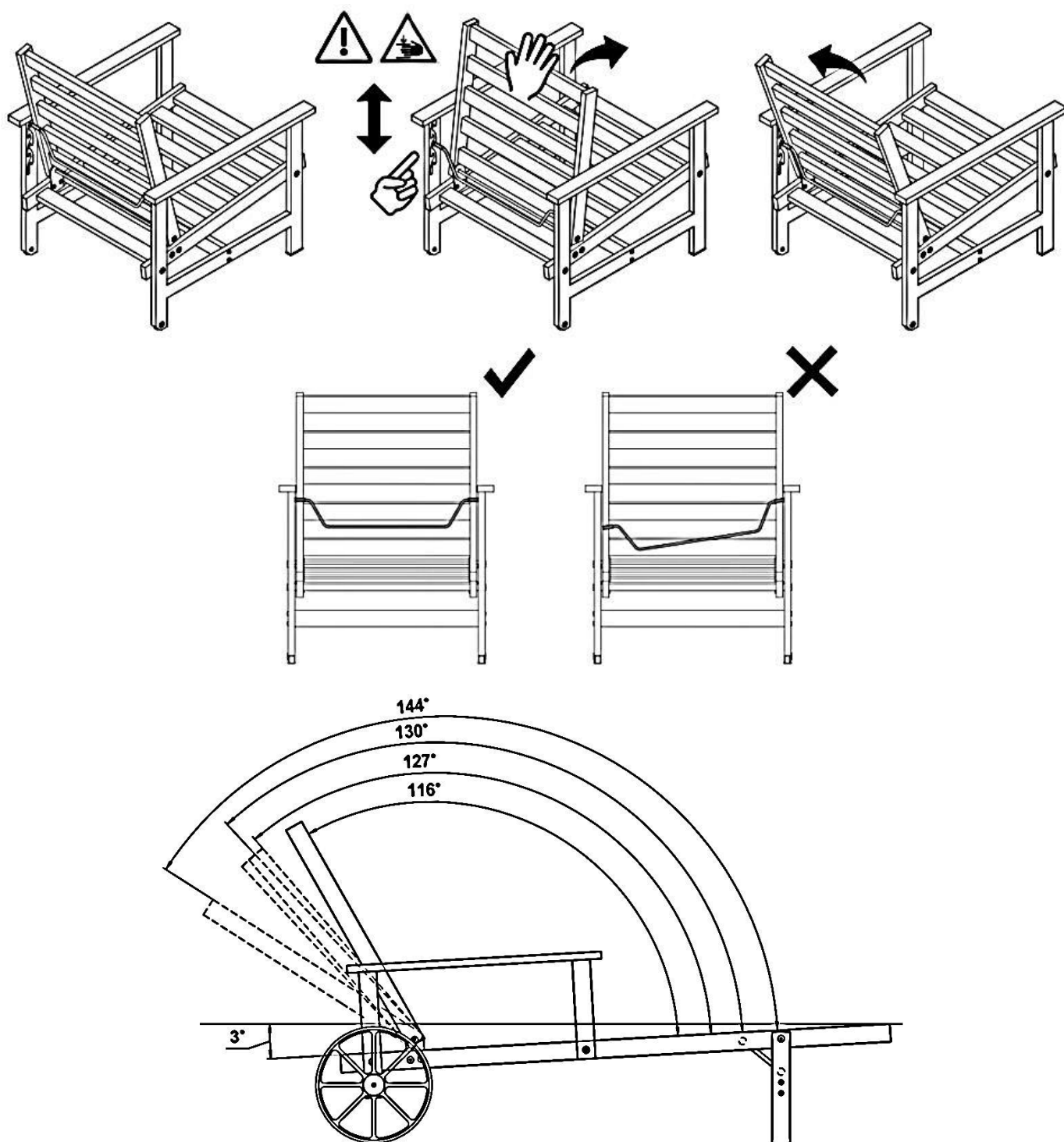
Рисунок 3 - Схема регулировки спинки изделий
